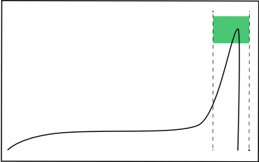
Drehmoment-/Winkelsteuerung
